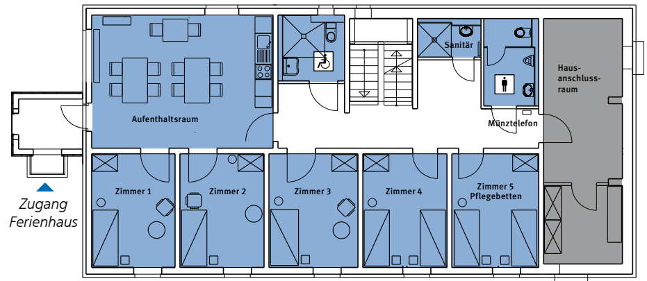
Grundriss Erdgeschoss
